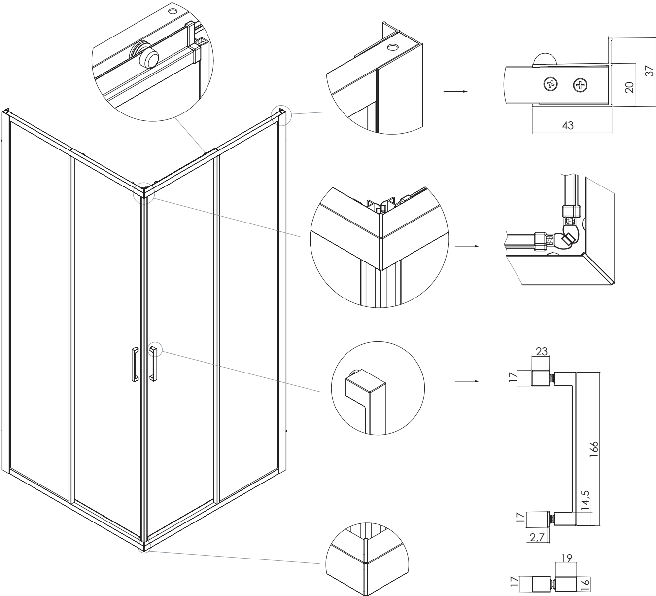
MISURE DISEGNO TUTTE IN MM
