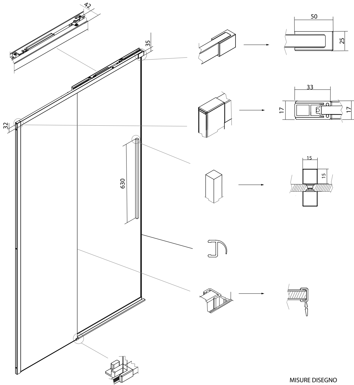
MISURE DISEGNO TUTTE IN MM
